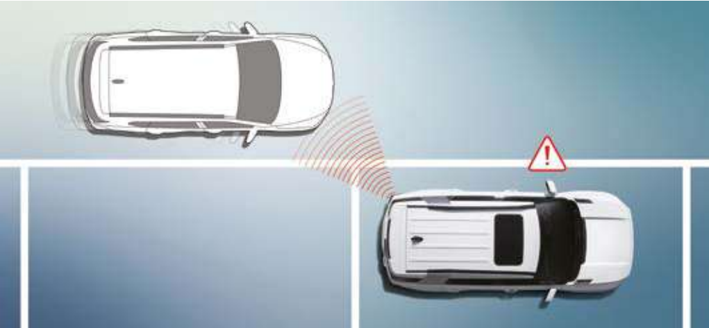
Sistema de salida segura del vehículo (SEW) Advierte del riesgo de colisión con vehículos situados en el ángulo muerto, cuando algún ocupante abre la puerta para salir del vehículo parado.
