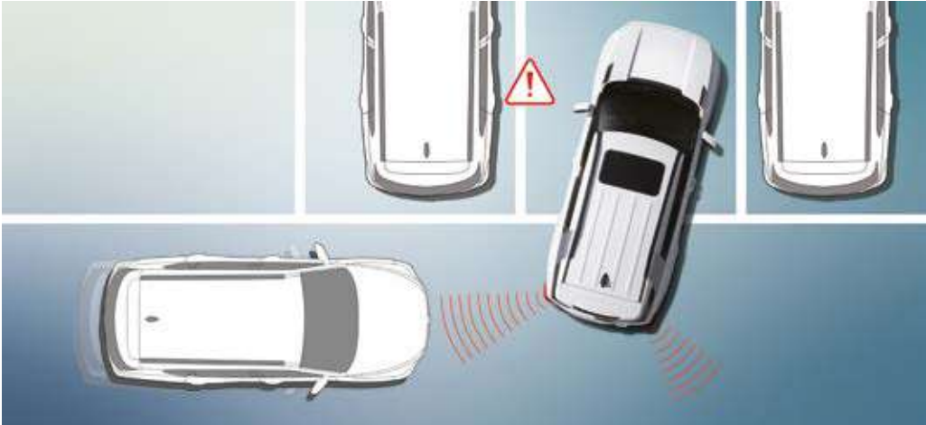
Sistema de alerta de tráfico trasero (RCTA) Al circular marcha atrás y detectar en la trayectoria un vehículo que se aproxima, el RCTA emite una alarma y acciona automáticamente los frenos para detener el vehículo y minimizar el riesgo de colisión.
