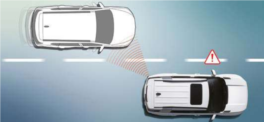
Control de ángulo muerto (BSD) Asiste automáticamente la frenada si, al cambiar de carril, se detecta riesgo de colisión con vehículos en el ángulo muerto.
