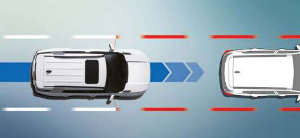
Sistema de permanencia en carril (LKAS) Sistema de advertencia de salida de carril (LDWS) El LKAS utiliza una cámara frontal para monitorizar las líneas pintadas de delimitación de carril. Al detectar un intento de cambio de carril sin señalización previa, corrige automáticamente la dirección asistida eléctrica para mantener el vehículo dentro del carril.
